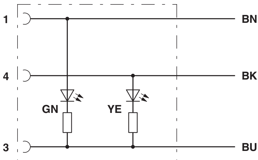
Affectation des contacts du connecteur femelle M12
