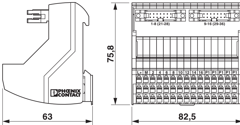
Maßzeichnung
