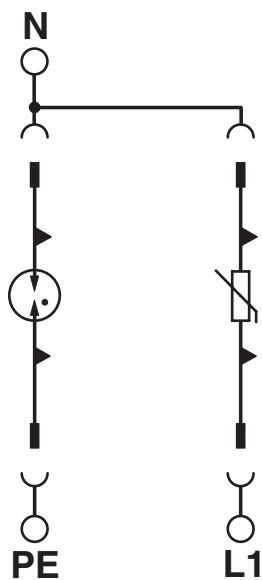
Diagrama eléctrico
