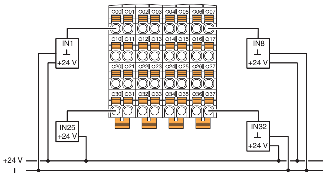
Conexión en tecnología de 1 conductor
