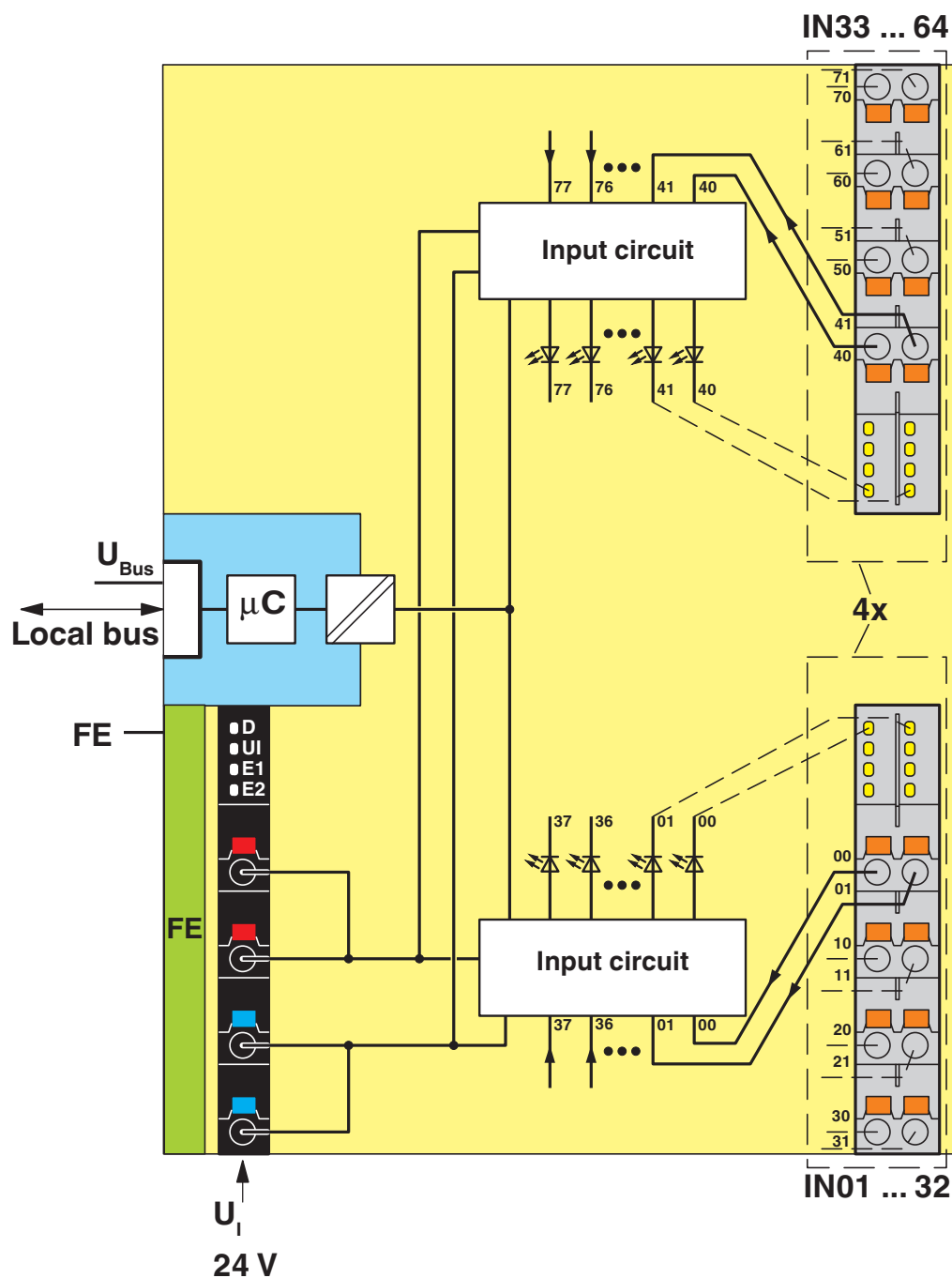
Schéma fonctionnel
