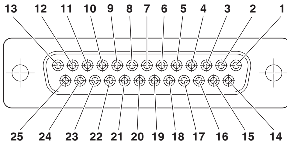
Plano esquemático
