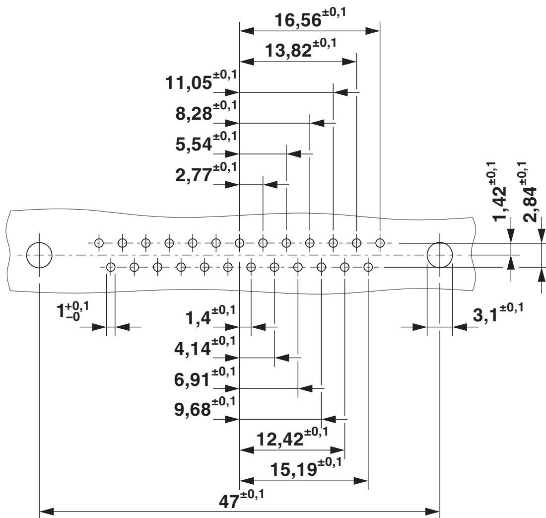
Gabarit perçage / géom. pastille soudage
