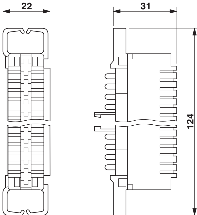
Maßzeichnung
