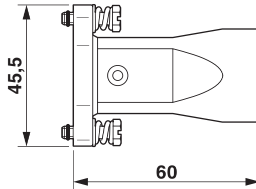
Maßzeichnung
