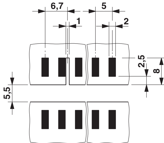
Esquema de taladros/geometría pads soldadura
