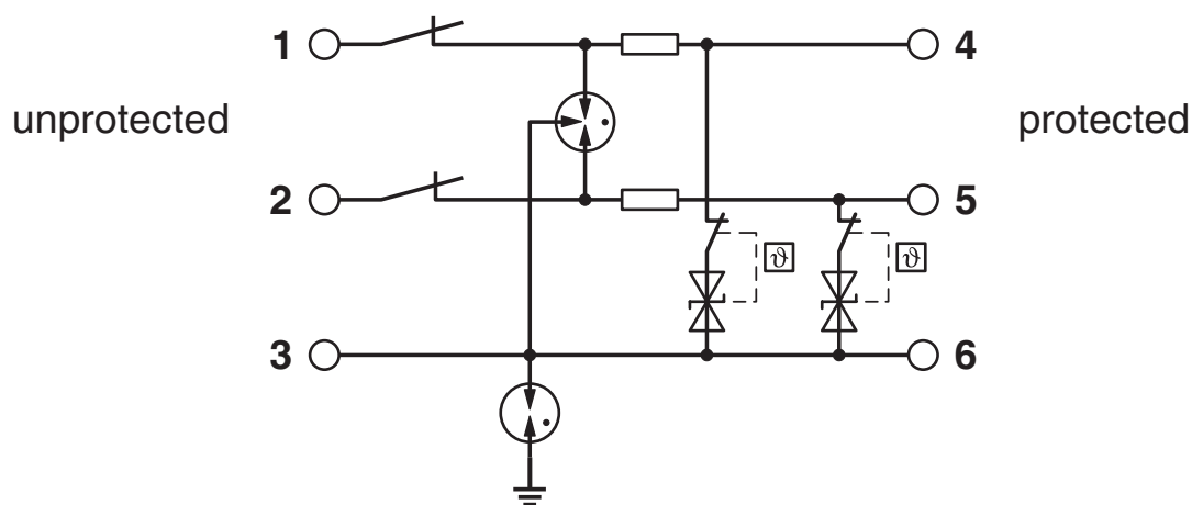
Diagrama eléctrico
