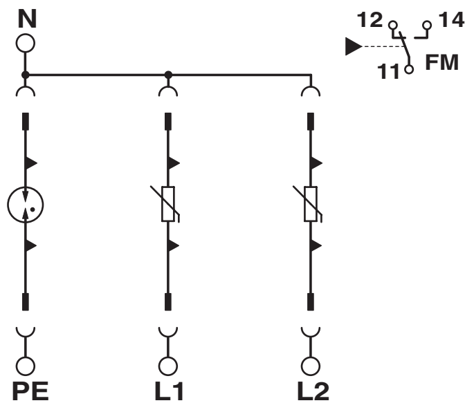
Schaltplan
