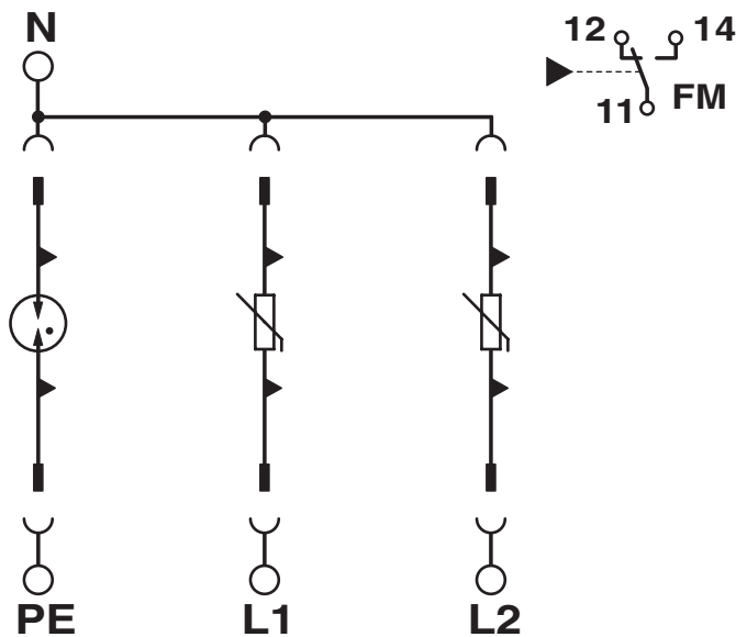
Diagrama eléctrico
