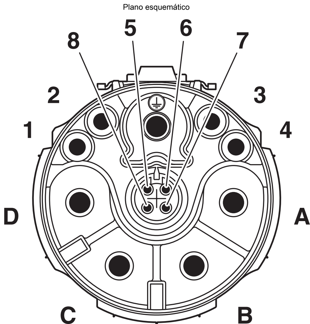
Esquema de polos conector macho señal, codificación 2
