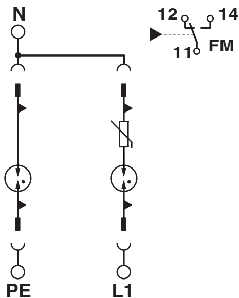
Schaltplan
