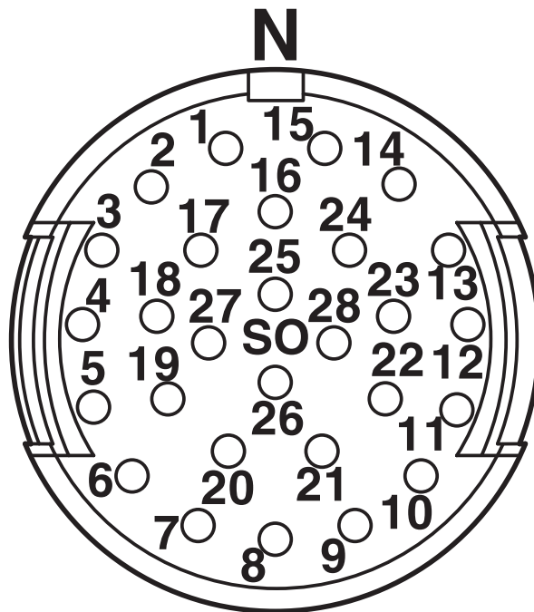
Schemazeichnung
