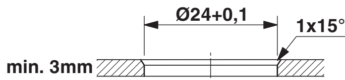
Dessin coté
