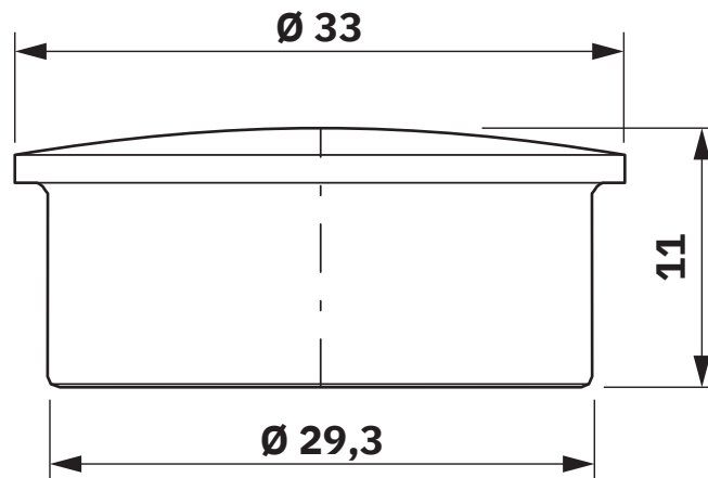
Maßzeichnung
