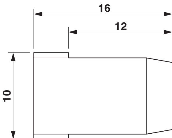
Maßzeichnung
