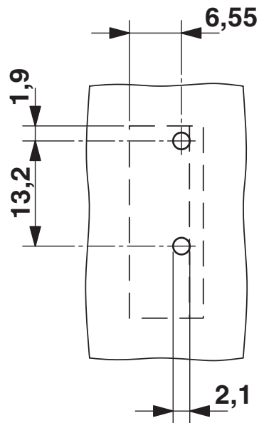
Bohrplan/Lötpadgeometrie
