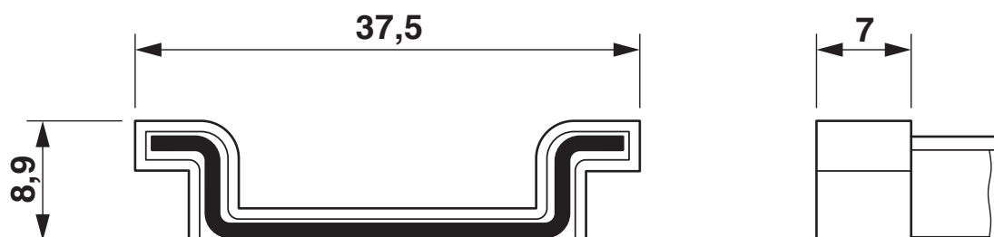
Dessin coté
