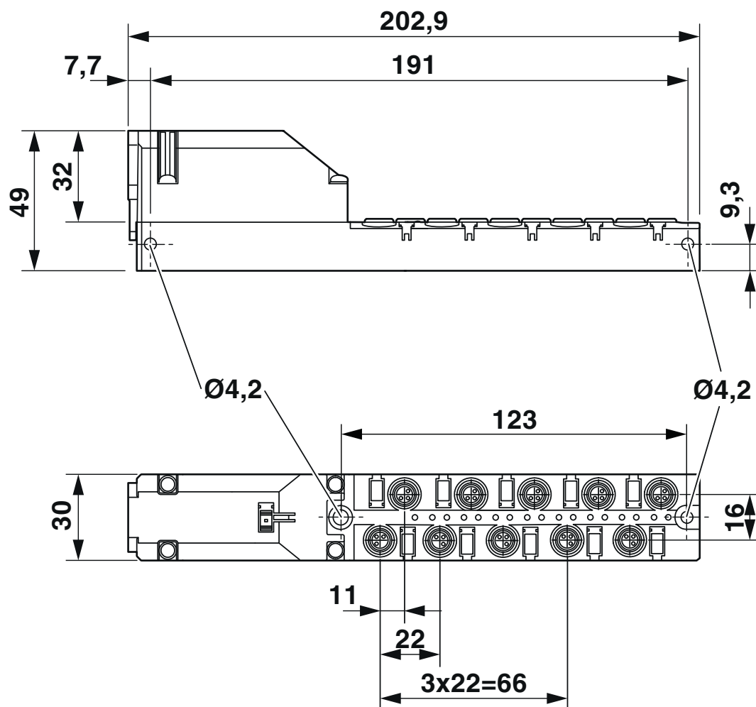
Dessin coté
