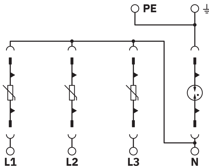
Diagrama eléctrico
