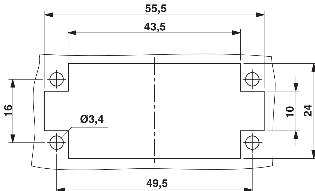
Montageausschnitt bei Verwendung ohne Gehäuse
