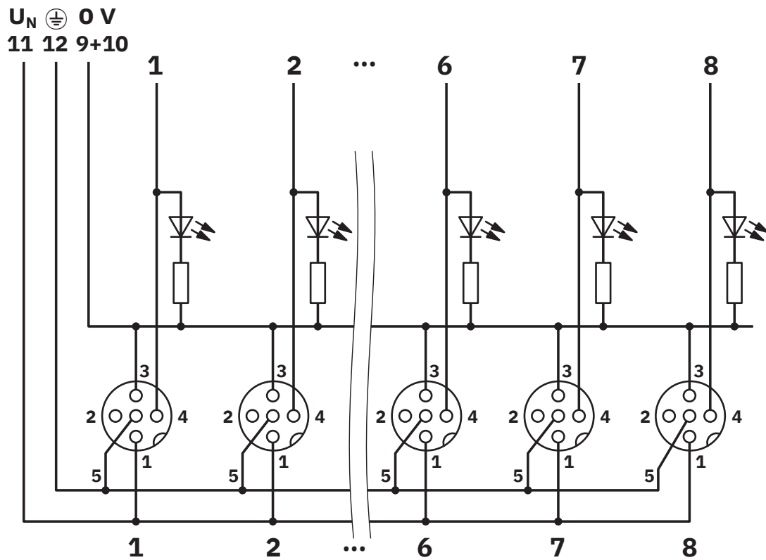
Diagrama eléctrico
