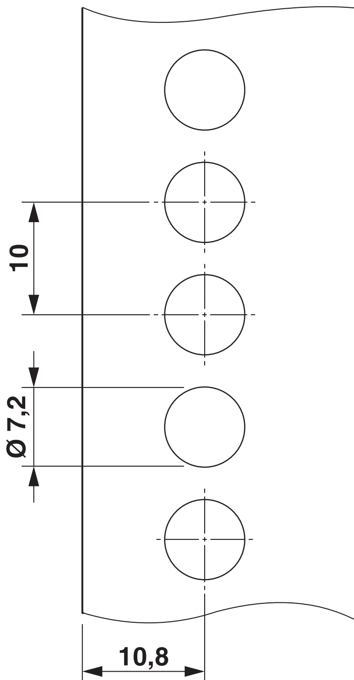
Esquema de taladros/geometría pads soldadura
