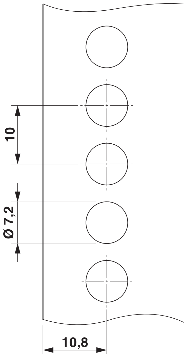
Gabarit perçage / géom. pastille soudage
