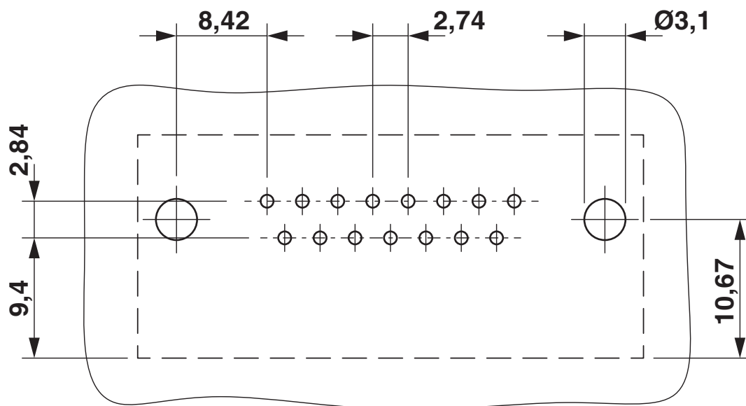
Bohrplan/Lötpadgeometrie
