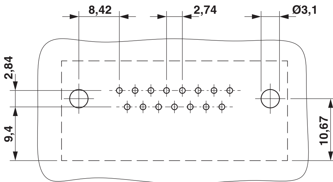
Gabarit perçage / géom. pastille soudage
