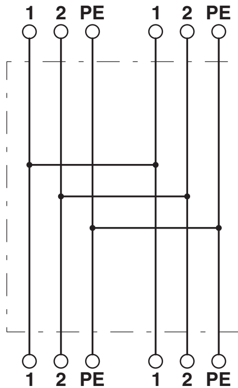
Schaltplan
