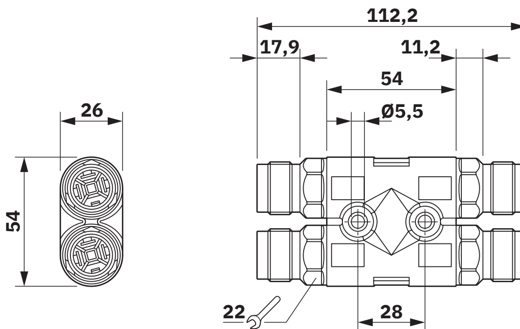
Dessin coté
