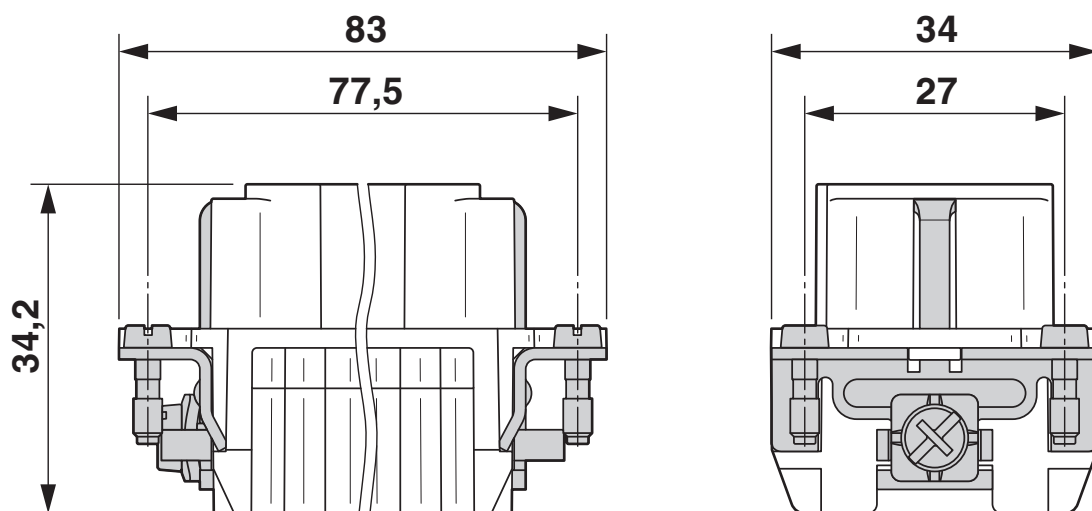
Maßzeichnung
