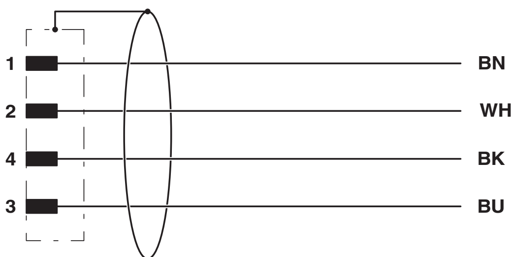
Diagrama eléctrico
