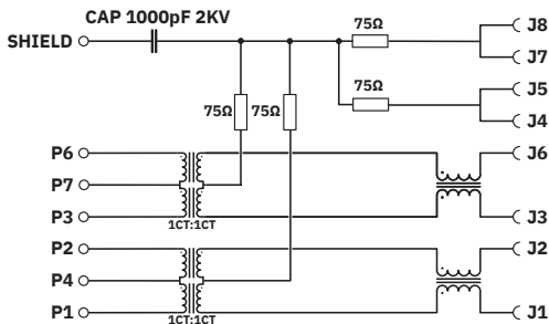
Schaltplan
