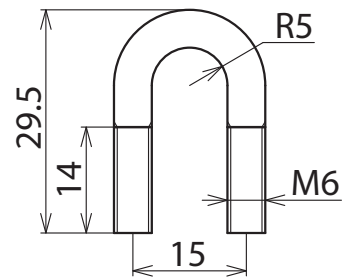
Maßbild MPE S 35 ER
