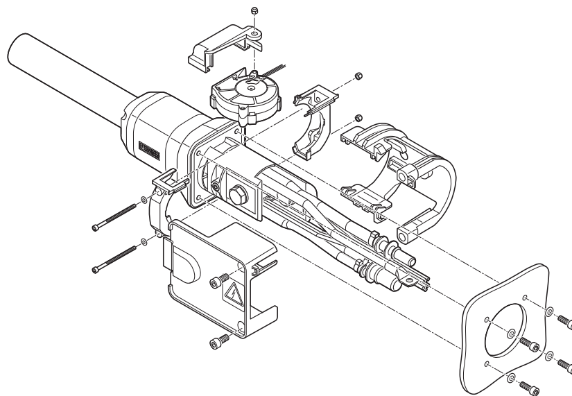
Dessin schématique
