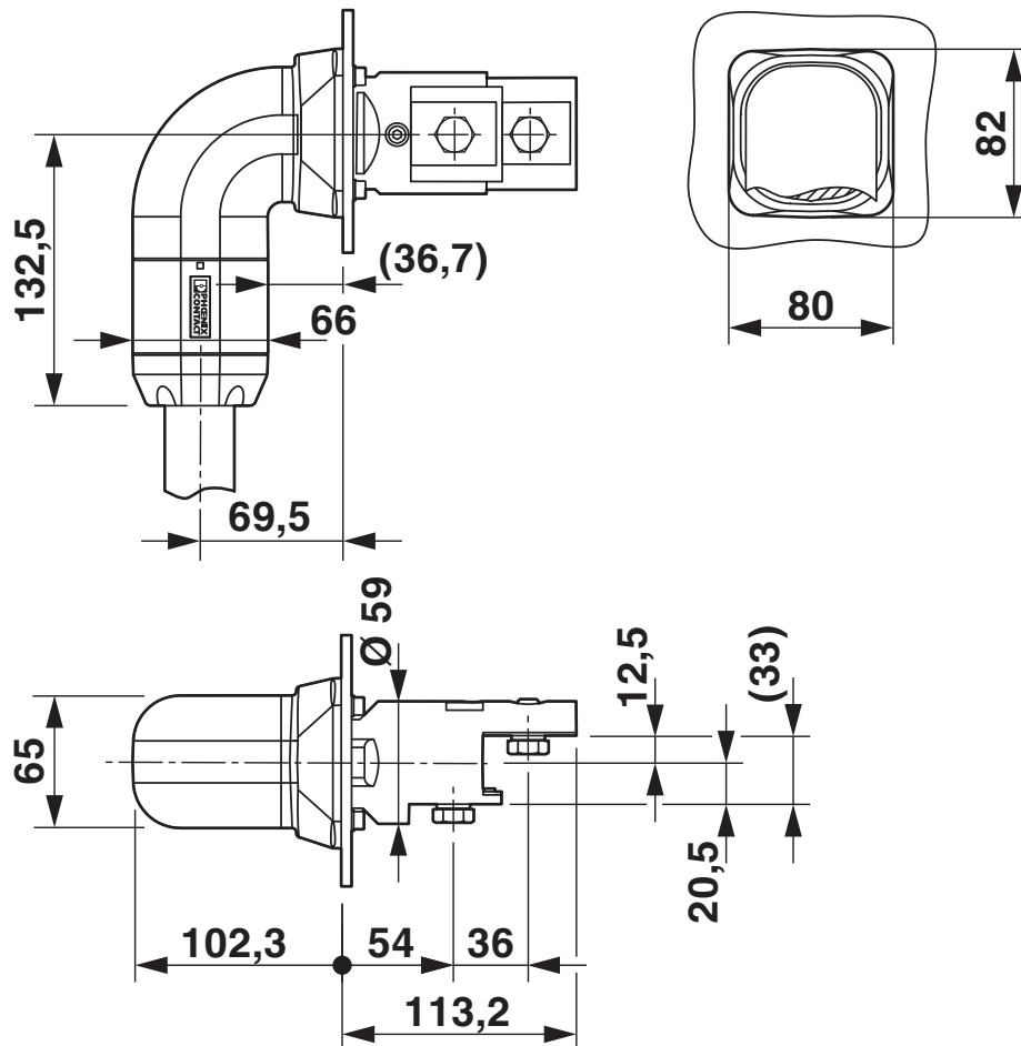
Dessin coté
