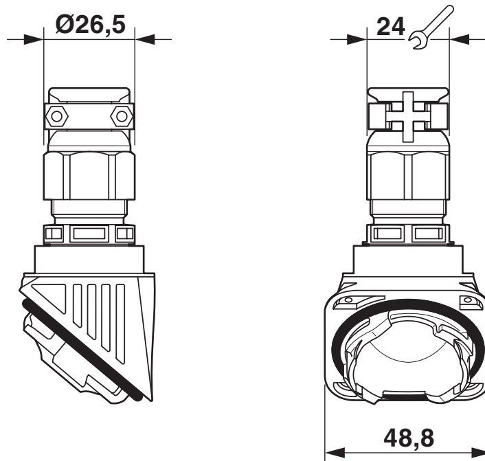
Dessin coté
