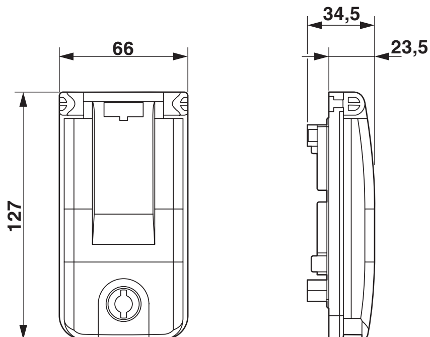
Dessin coté
