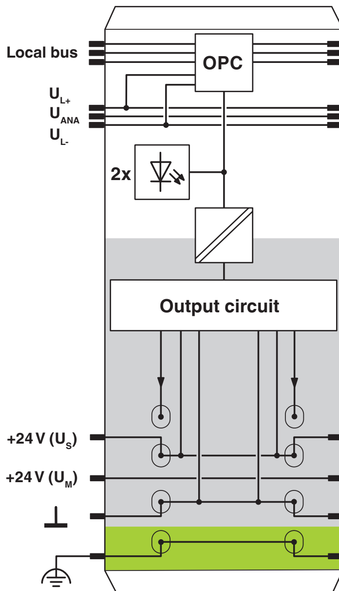
Schéma fonctionnel
