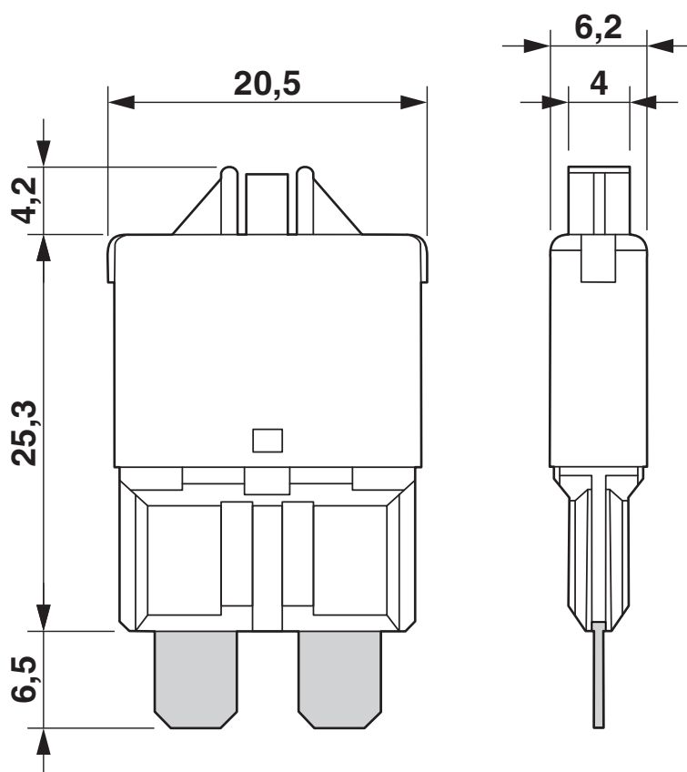
Dessin coté
