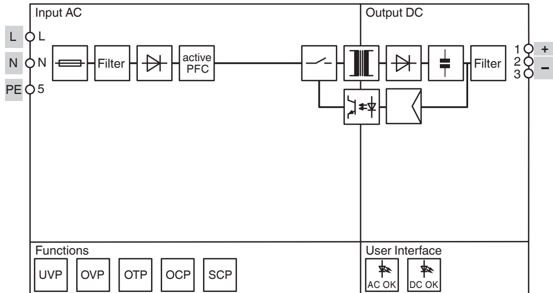
Blockschaltbild
