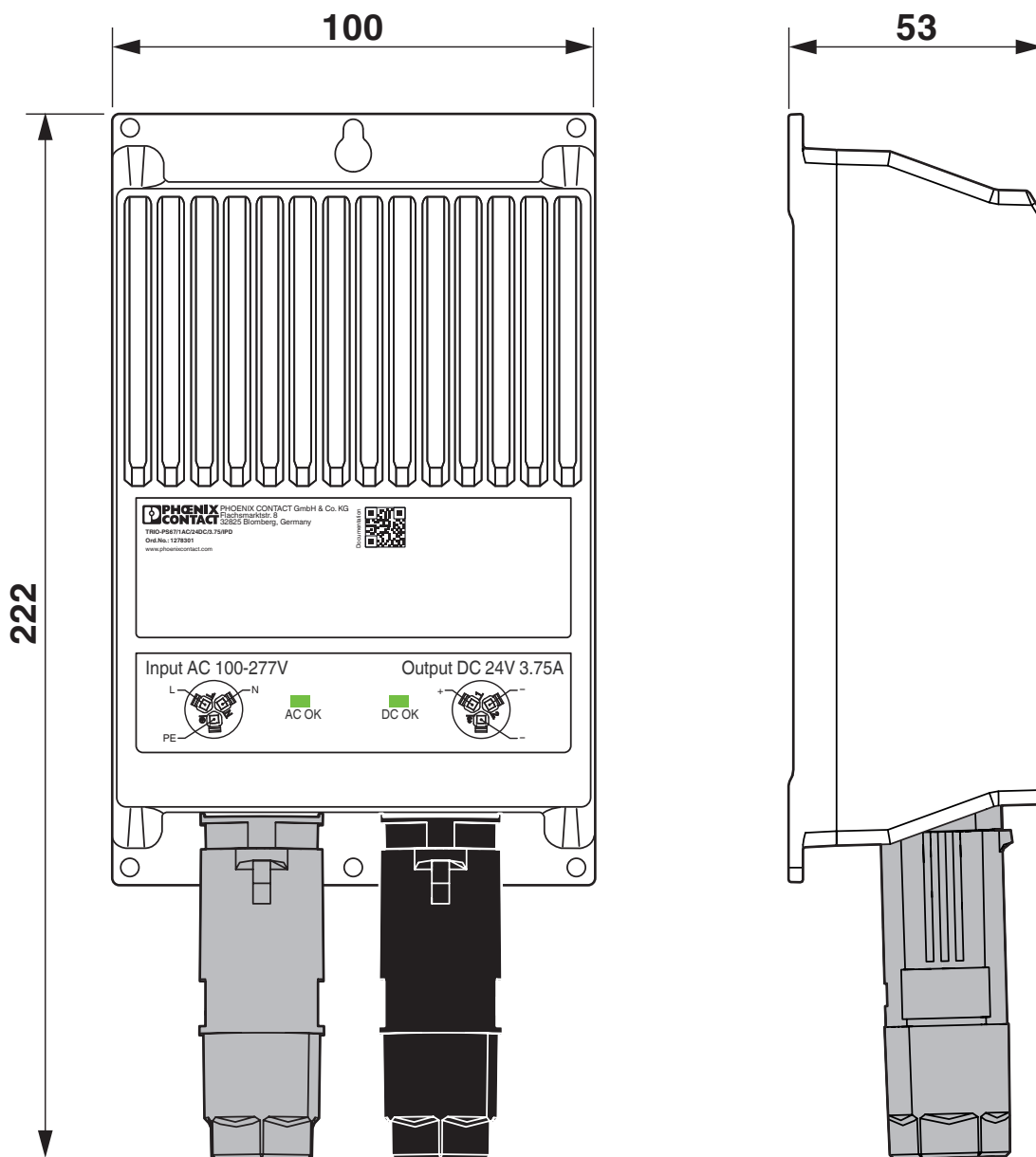
Maßzeichnung
