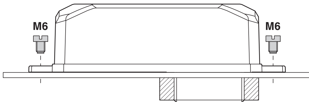
Schemazeichnung
