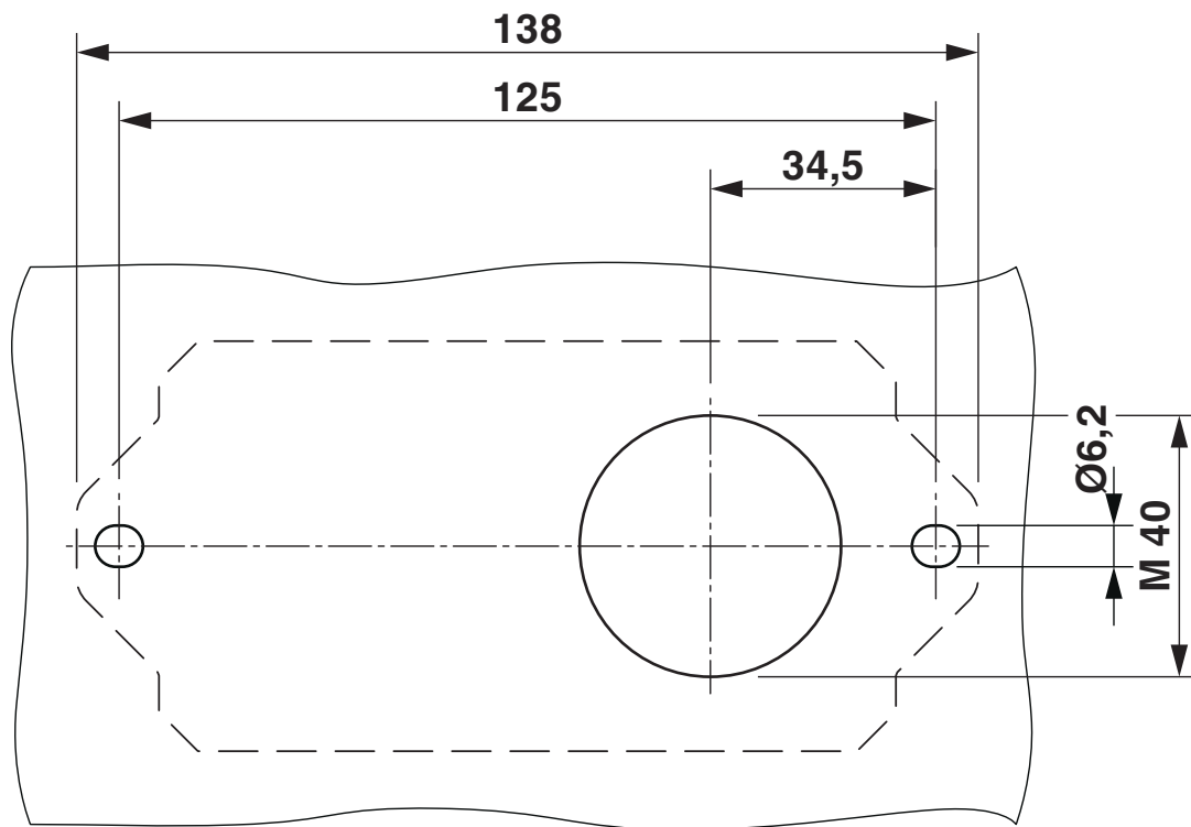
Maßzeichnung
