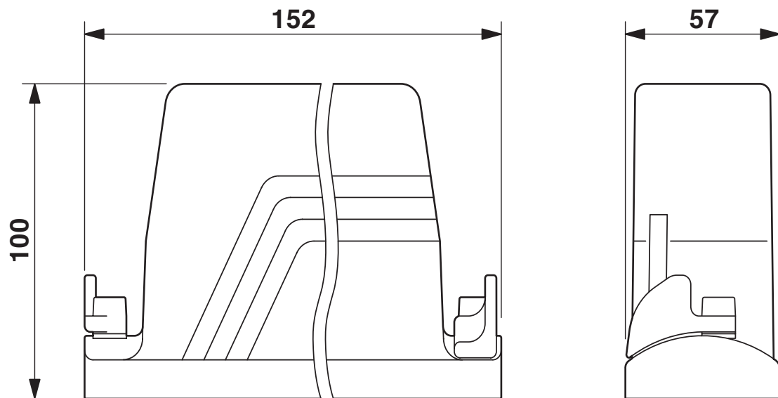
Maßzeichnung
