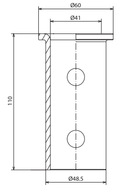
Maßbild AD 50 40 L110 STTZN
