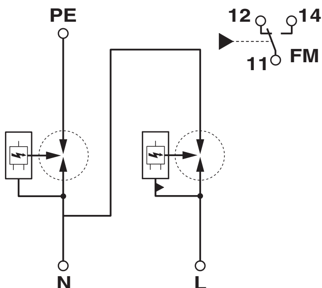
Diagrama eléctrico
