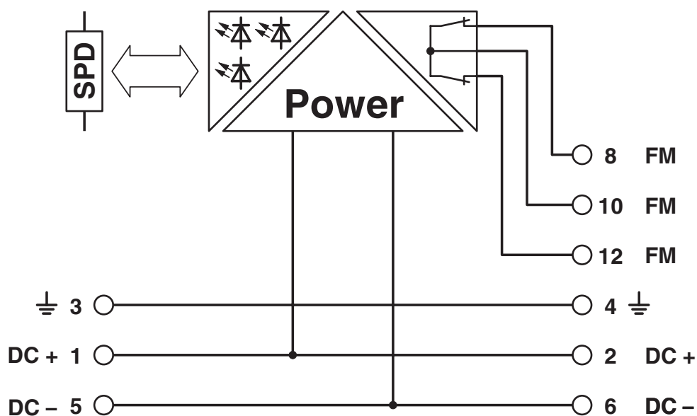
Diagrama eléctrico
