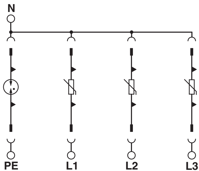
Schaltplan
