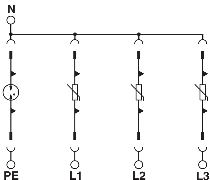
Diagrama eléctrico
