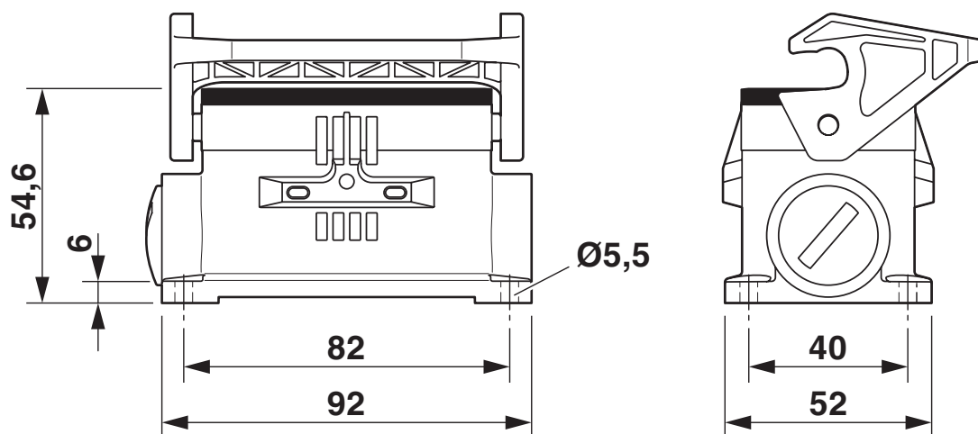
Dessin coté
