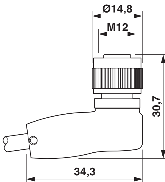
Dessin coté
